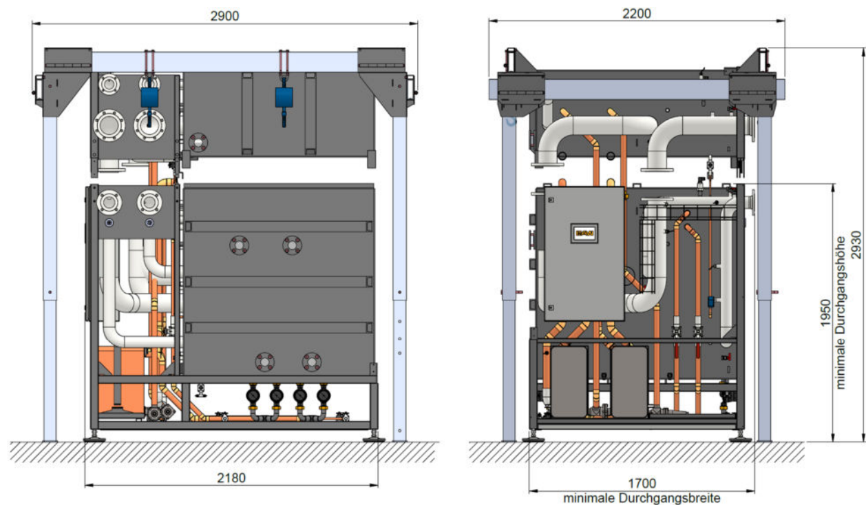
Abb.: Hebevorrichtung für Maral 5
